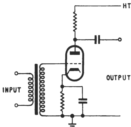
Fig. 1.47. Triode amplifier
