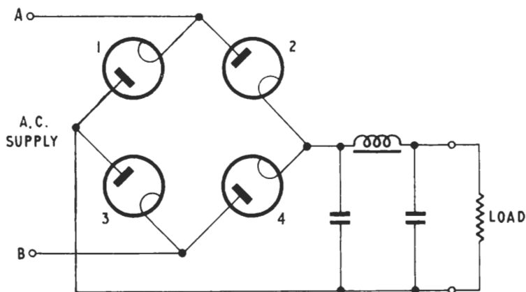
Fig. 1.45. Bridge rectifier
