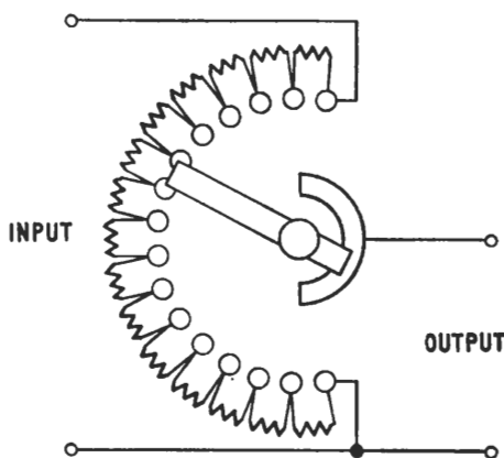
Fig. 1.23. Stud-type fader
